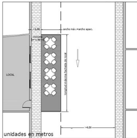
PLANTA 2 - ACERAS <3,00m
