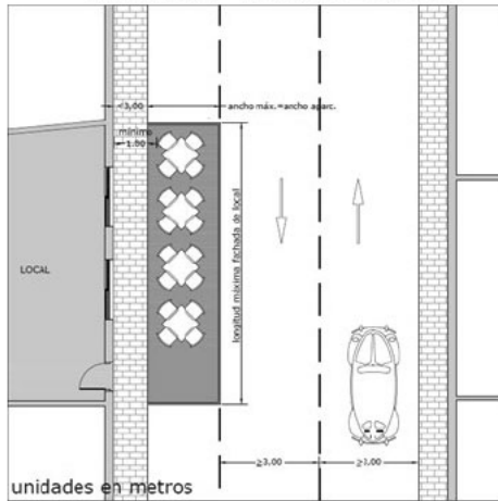
PLANTA 1 - ACERAS <3,00m
