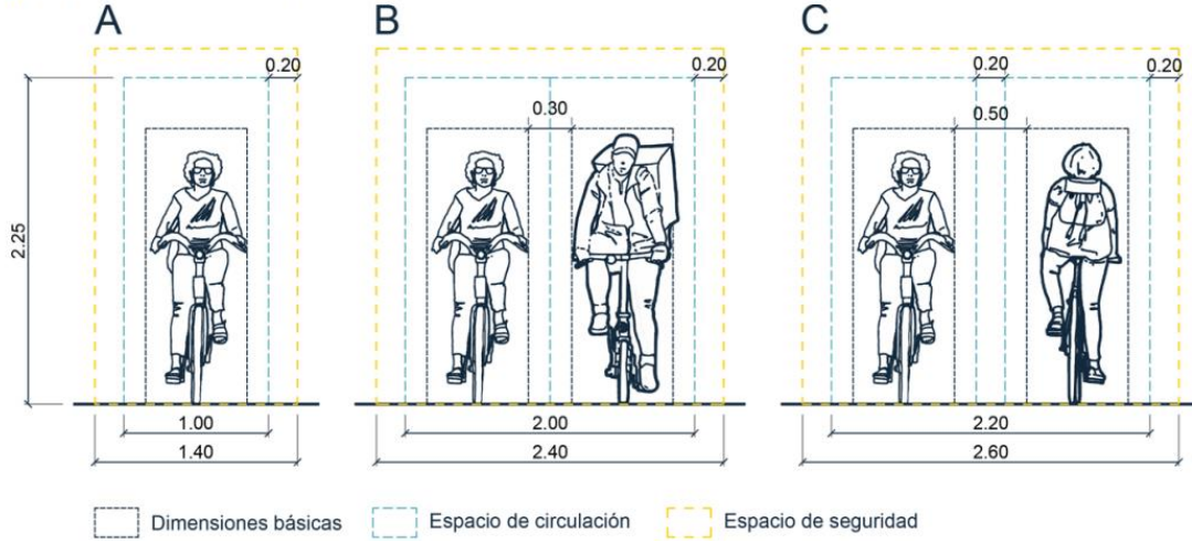
Figura 3.7 Dimensiones básicas del ciclista circulando
