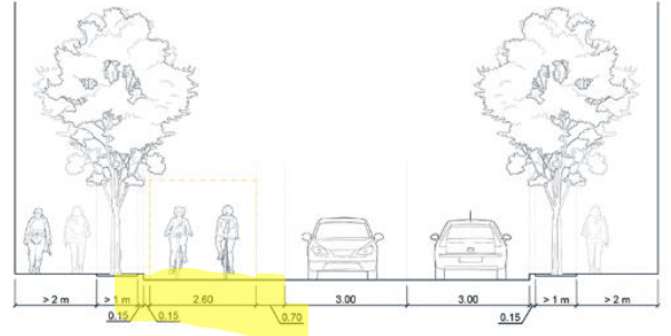
Figura 4.14 Esquema de vía ciclista bidireccional en lateral entre calzada y acera
