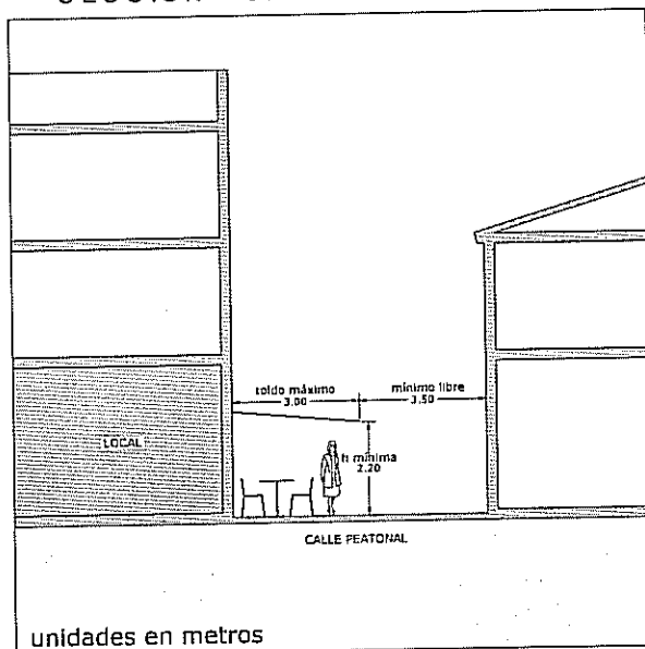
SECCIÓN - CALLE PEATONAL
